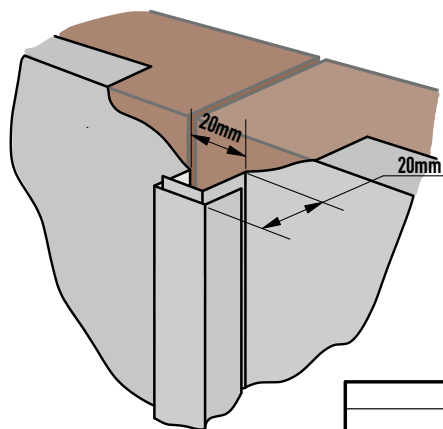
«усиленное» замковое соединение *
