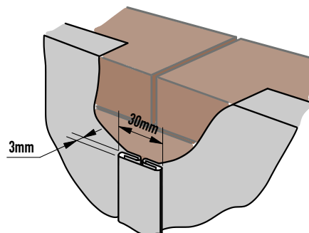
«цельное» замковое соединение*
