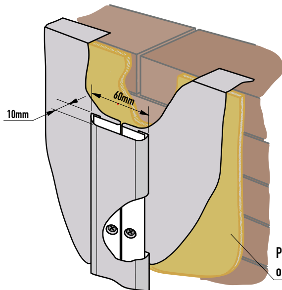
«разборное» замковое соединение *
